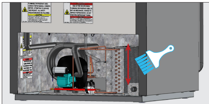
Rys. 3. Nigdy nie należy czyścić szczotką węzownicą w poprzek uźebrowania.
