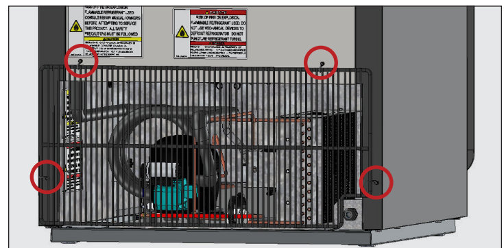
الشكل 2. أماكن براغي الشبكة الخلفية CVM-20/24/27.
