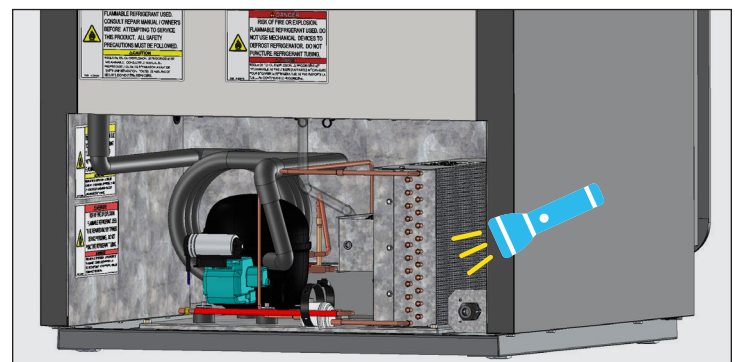
الشكل 4. تحقق من إزالة جميع الانسدادات.
